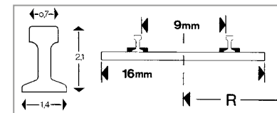
14975 Vario Gleis Vario Track Voie droite Rechte rail 312,6 mm
