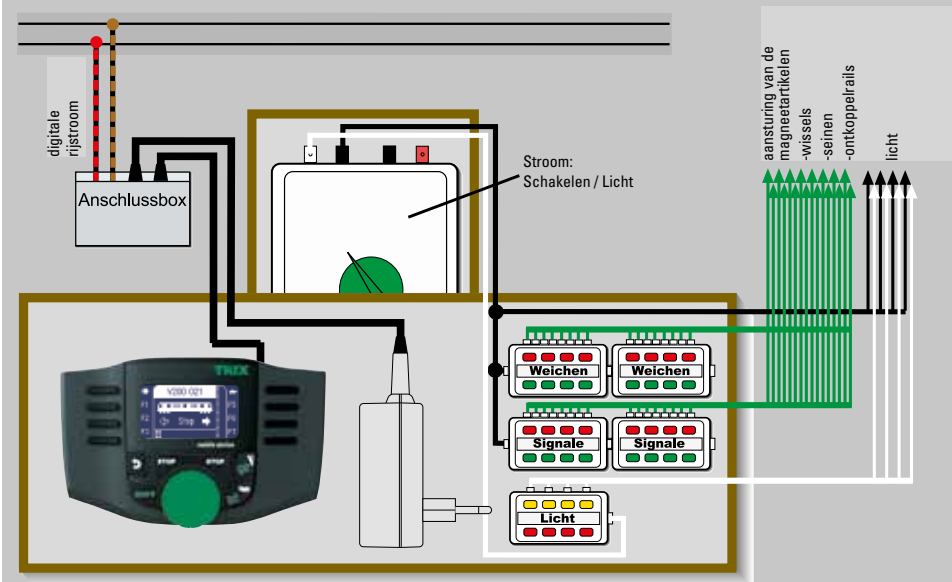
Digitaal besturen en schakelen met Trix Mobile Station en een schakelkastje voor de lichtstroom
