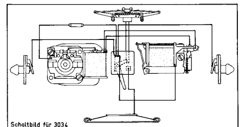
Schaltbild für 3034
