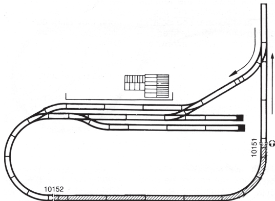
Bild 6 Gleisplanvorschlag
