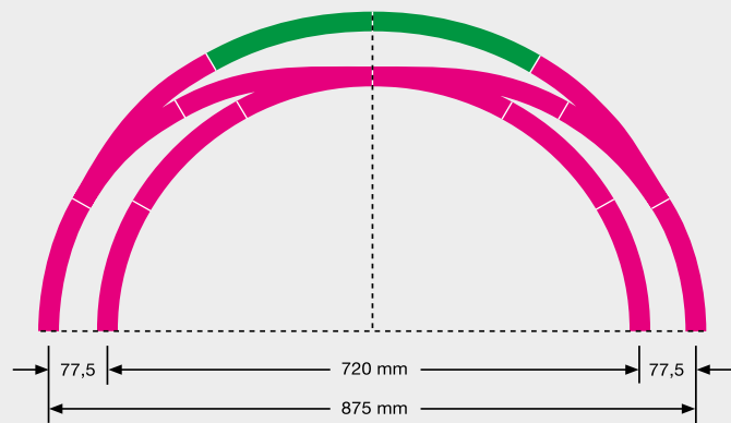
Bogenweichen mit runder Geometrie Curved Turnouts with Round Geometry Aiguilles enroulées Meegebogen wissels met ronde geometrie
