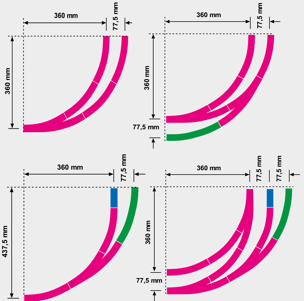
Bogenweichen mit runder Geometrie Curved Turnouts with Round Geometry Aiguilles enroulées Meegebogen wissels met ronde geometrie
