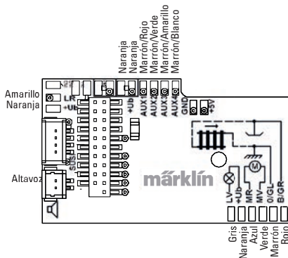
Designación Color de cable NEM Märklin Conexión de motor 2 gris azul Toma de corriente de 2 conductores vía izquierda Toma de corriente de 3 conductores vía exterior negro marrón Alumbrado de cabeza blanco gris Aux 1 verde marrón/rojo Conductor común para alumbrado/Aux 1 - 4 azul naranja Alumbrado de cola amarillo amarillo Toma de corriente de 2 conductores vía derecha Toma de corriente de 3 conductores vía centro rojo rojo Conexión de motor 1 naranja verde Aux 2 (salida física) violeta marrón/verde Aux 3 (salida física) marrón/ amarillo Aux 4 (salida física) marrón/ Blanco
